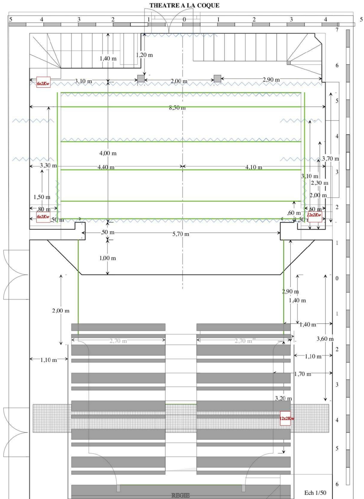
Plateau (plan avec cotes).
